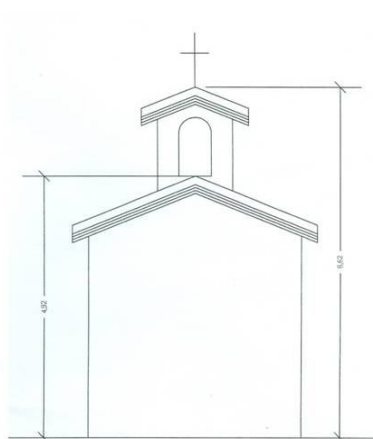
ALZADO POSTERIOR
